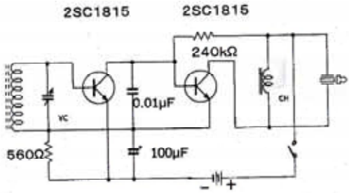
2石トランジスタラジオ回路図
